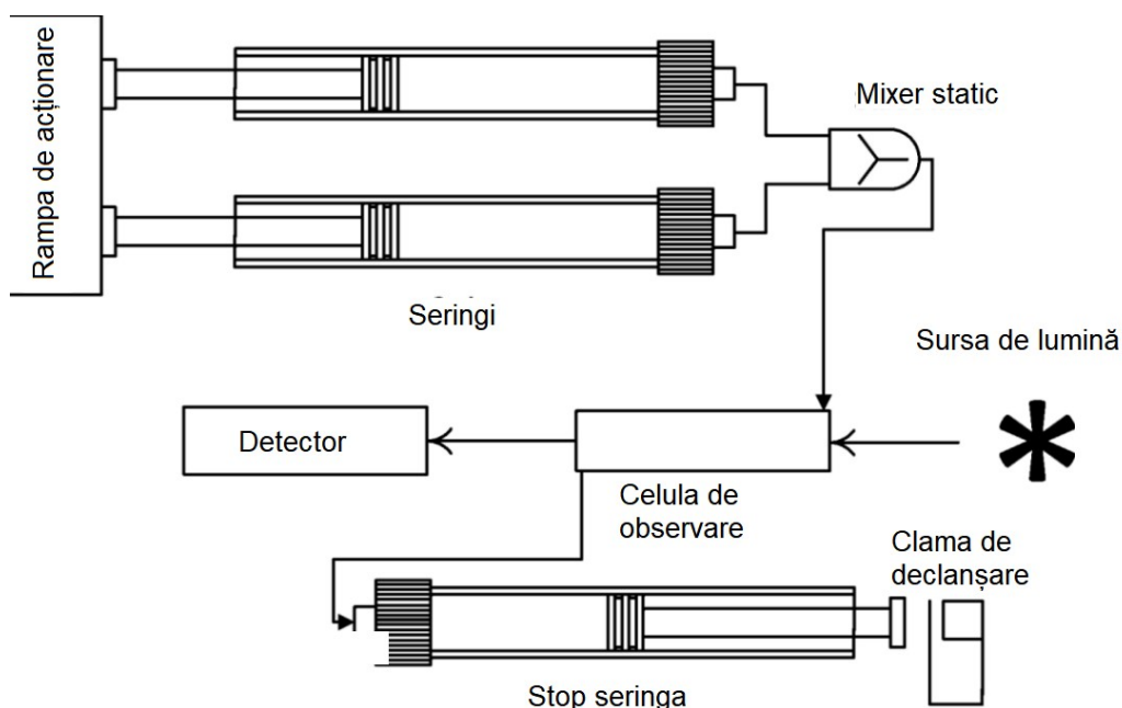
Fig. 2.4. Reprezentarea grafică a principiului de lucru al aparatului stopped-flow
