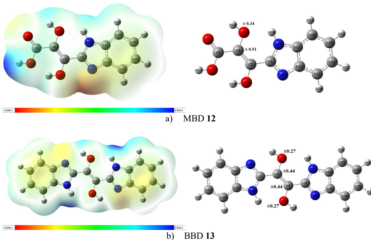
Fig. 4.9. Hărțile MEP (pe stânga) și indicele ambifilic R_k (pe dreapta) ale MBD 12 și BBD 13, în metanol
