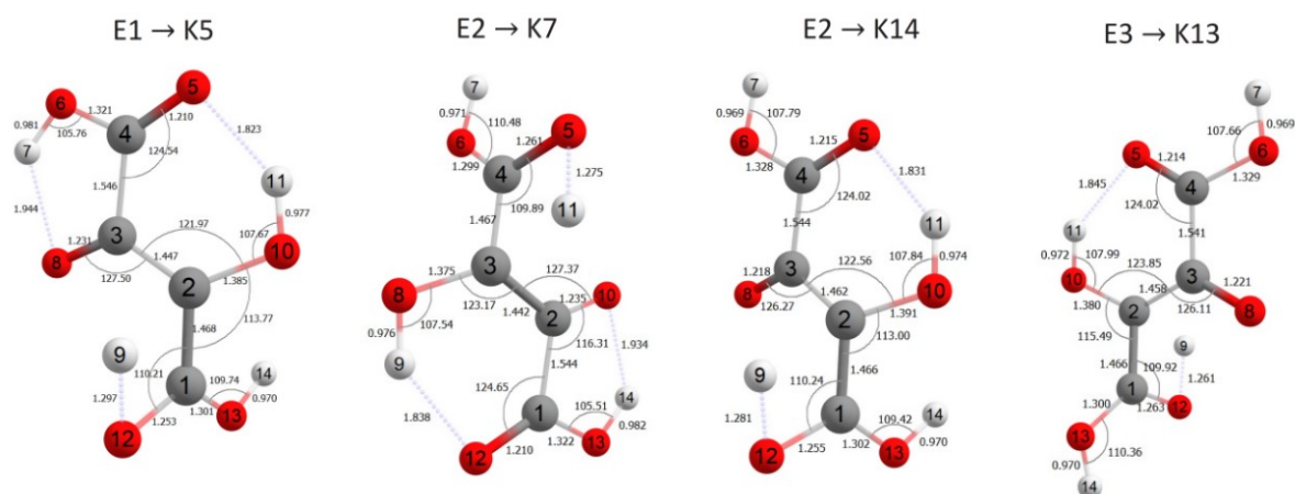
Fig. 4.5. Structurile geometrice optimizate ale stărilor de tranziție în tautomeria ceto-enolică a celor mai stabili trei izomeri ai DFH 4 , în vid.
