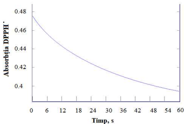
Fig. 3.25. Scăderea absorbției radicalului DPPH • în timp, la interacțiunea cu esterul 2 , în primele 60 de secunde de reacție, pentru condiția [EMD]_0 = [DPPH^{\bullet}]_0/\sigma , unde \sigma = 0.7
