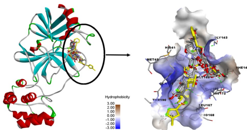
Figura 4.19. Poziția celei mai bune conformații pentru toți compușii studiați în buzunarul de legare al M pro al SARS-CoV-2 (ligandul co-cristalizat N3 este prezentat cu galben)
