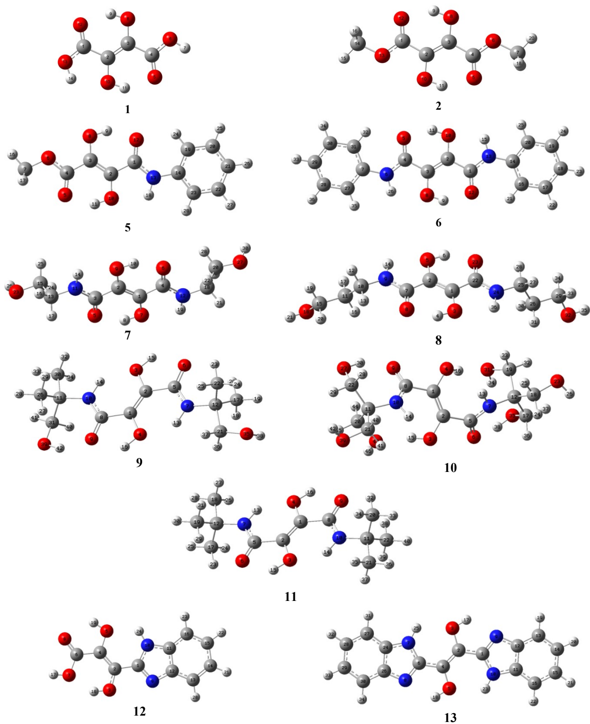
Fig. 4.6. Structurile optimizate ale compușilor cercetați în soluție apoasă: 1 - DFH 4 , 2 - dimetil 2,3-dihidroxifumarat, 5 - ( E )-metil 2,3-dihidroxi-4-oxo-4-(fenilamino)but-2-enoat, 6 - 2,3-dihidroxi-N1,N4-di(piridin-2-il)fumaramida, 7 - MEAD, 8 - MPAD, 9 - 2,3-dihidroxi-N1,N4-bis(1-hidroxi-2-metilpropan-2-il)fumaramida, 10 - N1,N4-bis(1,3-dihidroxi-2-(hidroximetil)propan-2-il)-2,3-dihidroxifumaramida, 11 - N1,N4-di-tert-butil-2,3-dihidroxifumaramida, 12 - MBD, 13 - BBD
