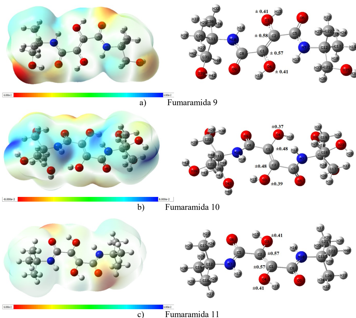
Fig. 4.11. Hărțile MEP (pe stânga) și indicele ambifilic R_k (pe dreapta) ale fumaramidelor 9 (a), 10 (b) și 11 (c), în metanol
