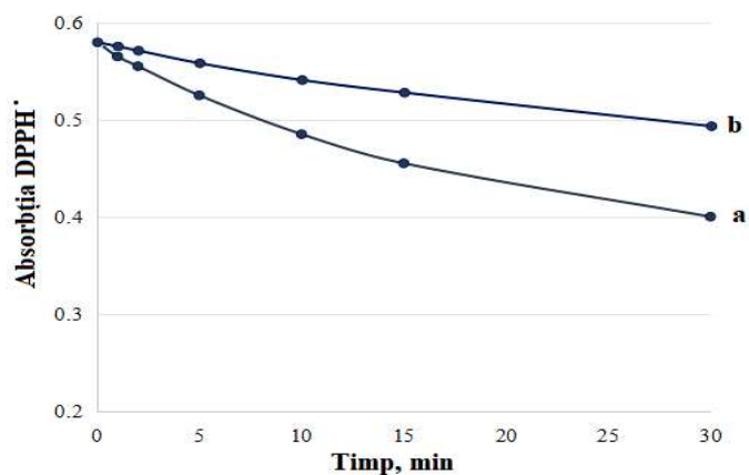
Fig. 3.13. Curbele cinetice de consum a DPPH' la interacțiunea cu: (a) anilida 5, [anilida]_0 = 2,26 \cdot 10^{-5} \text{ M} , [DPPH']_0 = 6 \cdot 10^{-5} \text{ M} , t = 30 \text{ min} și (b) fumaramida 6, [fumaramida]_0 = 2,7 \cdot 10^{-5} \text{ M} ; [DPPH']_0 = 6 \cdot 10^{-5} \text{ M} , t = 30 \text{ min}
