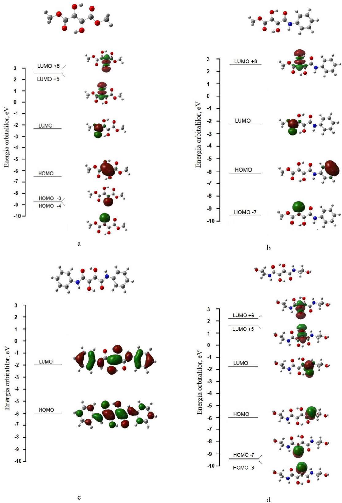
Fig. 4.14. Energia orbitalilor și unii orbitali moleculari de frontieră pentru (a) esterul EMD 2, (b) anilida 5, (c) fumaramida 6 și (d) MEAD 7
