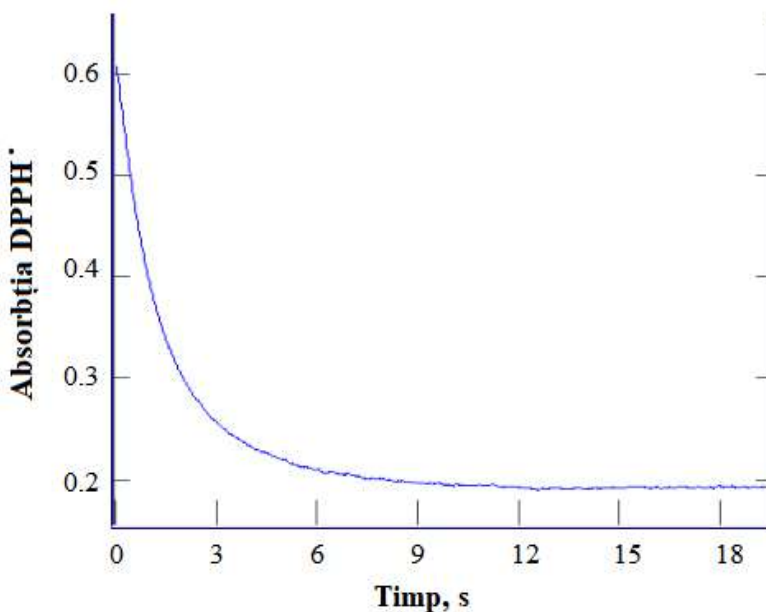
Fig. 3.17. Scăderea absorbției radicalului DPPH• în timp, la interacțiunea cu AAs, în primele 18 secunde de reacție, pentru condiția [AAs]_0 = [DPPH•]_0/\sigma , unde \sigma = 2
