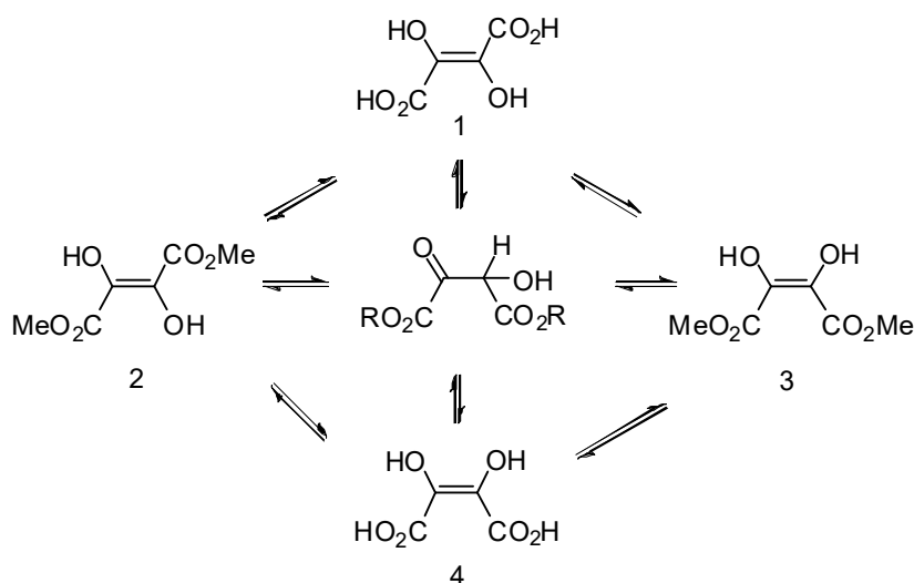
Fig. 3.2. Transformările formelor izomerice ale DFH 4
