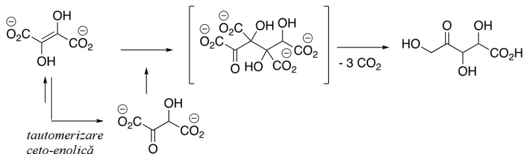
Fig. 1.13. Reprezentarea schematică a procesului de autocondensare a \text{DFH}_2^{2-} [58]
