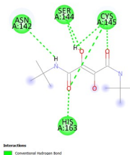
Fig. 4.22. Reprezentarea interacțiunii cu cel mai mare scor de andocare între compusul cercetat și proteaza principală a virusului SARS-COV-2 (imagine 3D - pe stânga și 2D - pe dreapta), pentru fumaramidele 9 (a), 10 (b) și 11 (c)
