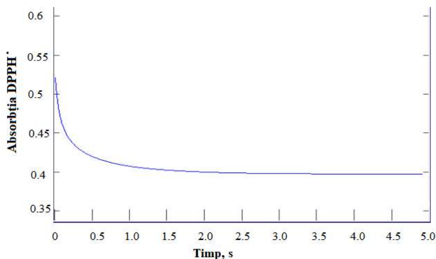
Fig. 3.21. Scăderea absorbății radicalului DPPH• în timp, la interacțiunea cu MBD 12, în primele 5 secunde de reacție, pentru condiția [MBD]_0 = [DPPH•]_0/\sigma , unde \sigma = 2
