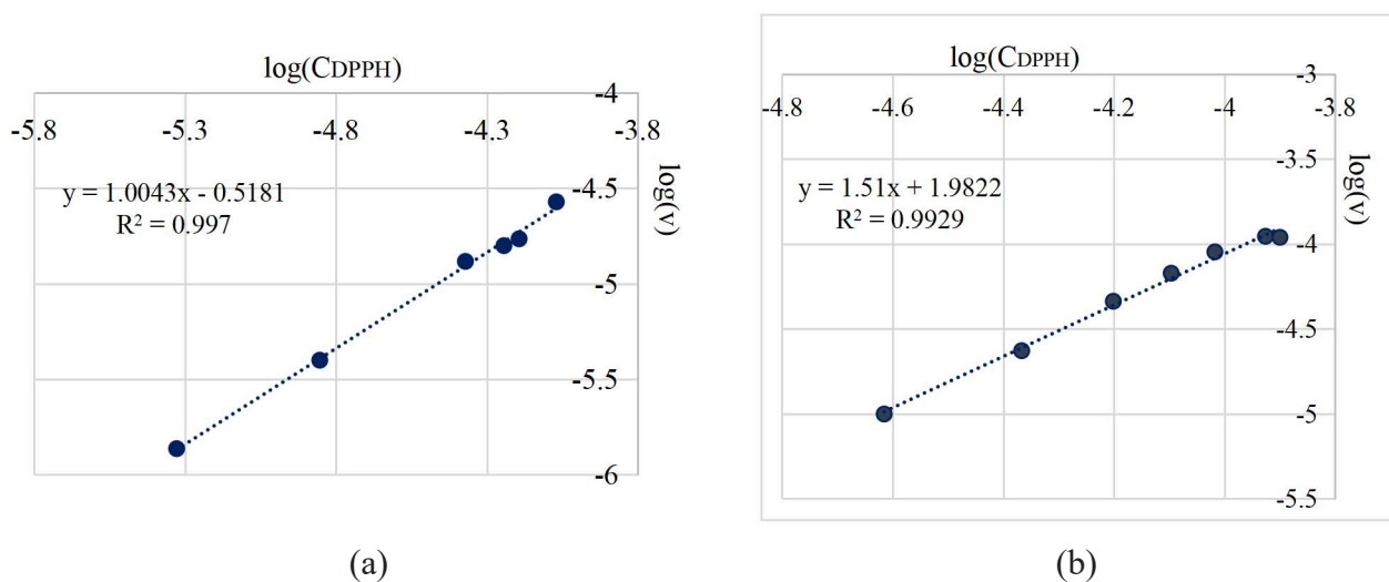
Fig. 3.20. Determinarea ordinului de reacție x față de DPPH• (a), și a ordinului total de reacție x+y (b) în reacția radicalului DPPH• cu DFH 4 1, unde [DFH_4]_0 = 2 \cdot 10^{-5} M (a) și [DFH_4]_0 = [DPPH^*]_0/\sigma (b), la timpul de reacție t = 0.3 s
