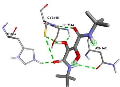
Fig. 4.22. Reprezentarea interacțiunii cu cel mai mare scor de andocare între compusul cercetat și proteaza principală a virusului SARS-COV-2 (imagine 3D - pe stânga și 2D - pe dreapta), pentru fumaramidele 9 (a), 10 (b) și 11 (c)
