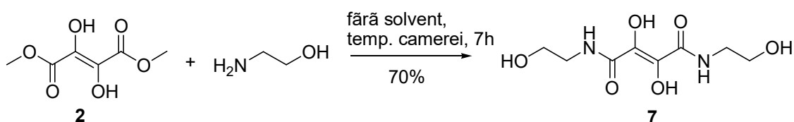
Fig. 3.5. Schema de sinteză a 2,3-dihidroxi-N1,N4-bis(2-hidroxietyl)fumaramidei 7
