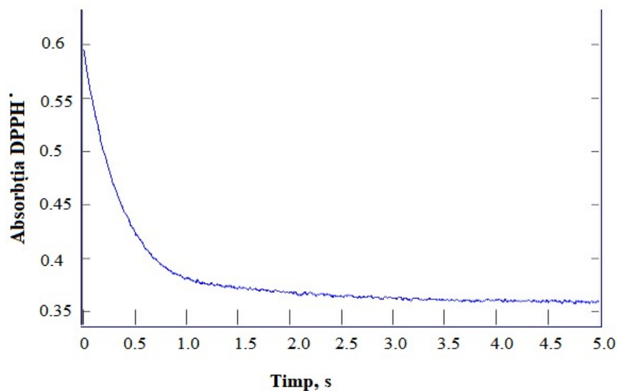
Fig. 3.19. Scăderea absorbății radicalului DPPH• în timp, la interacțiunea cu DFH 4 1, în primele 5 secunde de reacție, pentru condiția [DFH_4]_0 = [DPPH^*]_0/\sigma , unde \sigma = 2
