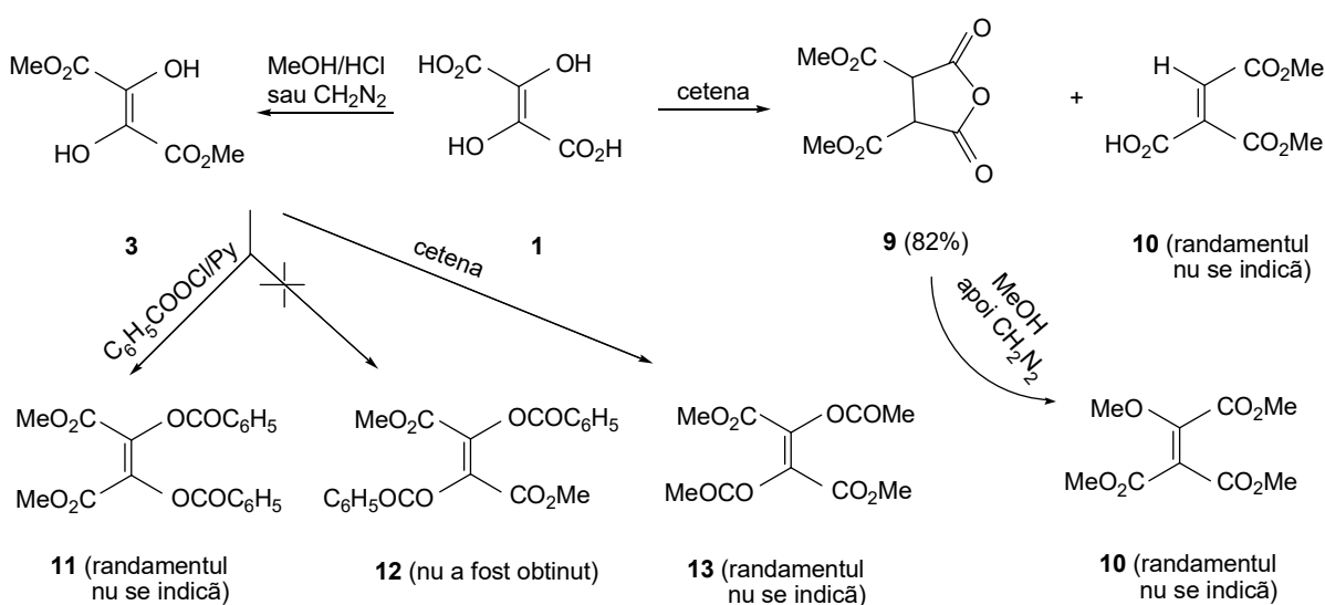
Fig. 1.5. Reprezentarea schematică a transformărilor chimice ale DFH 4 din [40]
