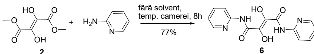
Fig. 3.4. Schema de sinteză a 2,3-dihidroxi-N1,N4-di(piridin-2-il)fumaramidei 6
