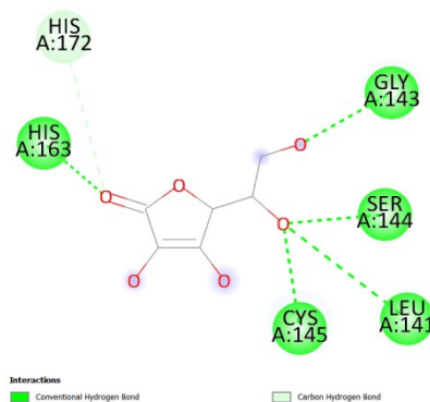
Fig. 4.20. Reprezentarea interacțiunilor cu cel mai mare scor de andocare între proteaza principală a virusului SARS-COV-2 și (a) acidul DFH 4 1, (b) esterul EDM 2, (c) acidul ascorbic (imagine 3D - pe stânga și 2D - pe dreapta)
