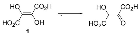
Fig. 1.1. Reprezentarea schematică a tautomeriei DFH 4
