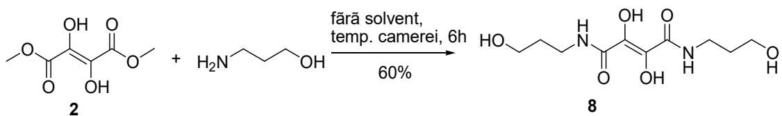
Fig. 3.6. Schema de sinteză a 2,3-dihidroxi-N1,N4-bis(2-hidroxiopropil)fumaramidei 8
