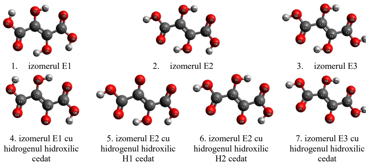
Figura 4.17. Speciile moleculare cu caracter antioxidant cercetate în solvent (apă).
