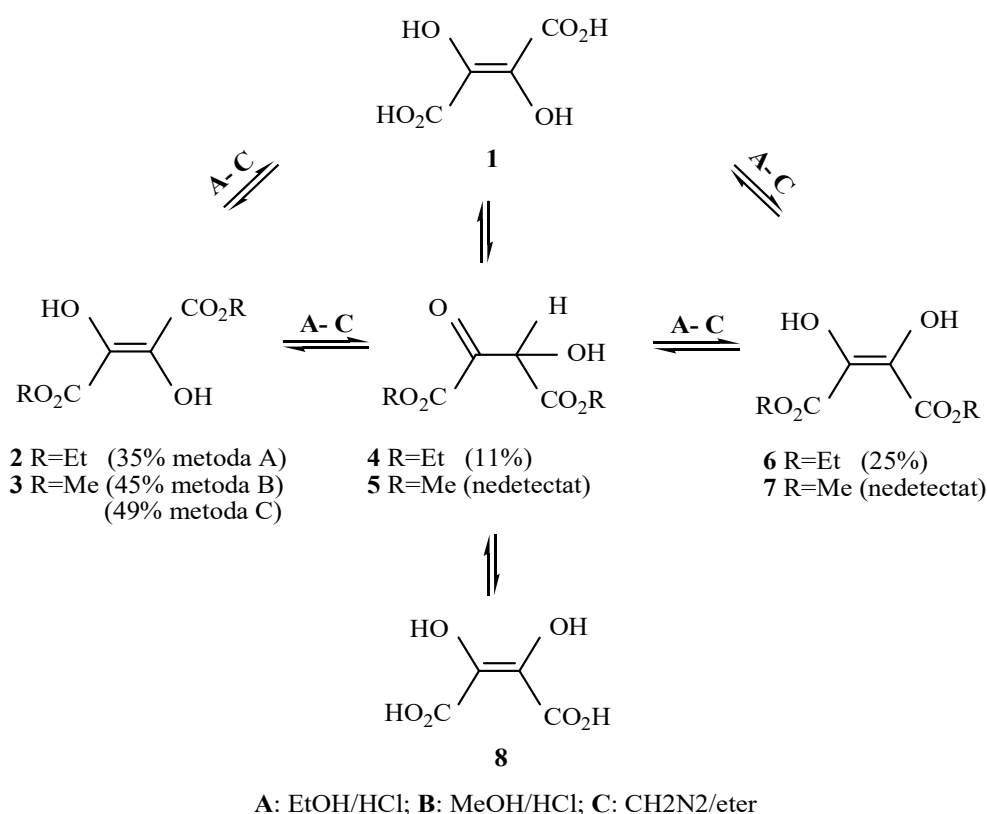
Fig. 1.4. Reprezentarea schematică a transformărilor chimice ale DFH 4 din [16]
