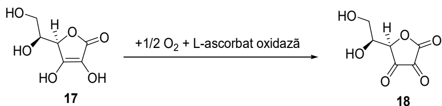
Fig. 1.9. Transformarea acidului ascorbic sub acțiunea L-ascorbat oxidazei
