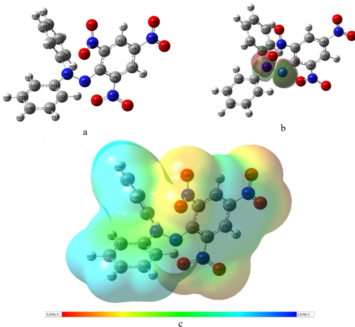
Fig. 4.16. Geometria optimizată a DPPH* (a), orbitalii moleculari \beta -LUMO +3 responsabili pentru acceptul electronului de la antioxidant (b) și harta potențialului molecular electrostatic (c)
