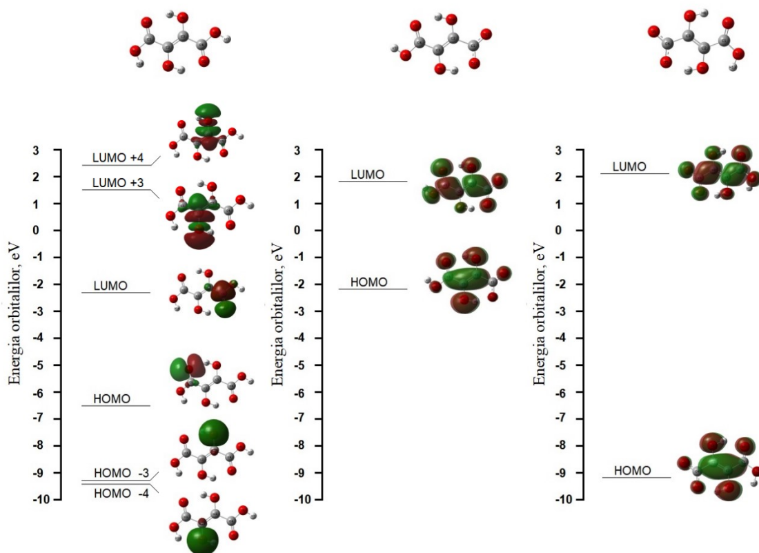
Fig. 4.12. Energia orbitalilor și unii orbitali moleculari de frontieră ai izomerului E2 (stânga) al acidului DFH 4 , anionul cu hidrogenul din poziția anti -disociat (centru) și anionul cu hidrogenul din poziția syn -disociat (dreapta)
