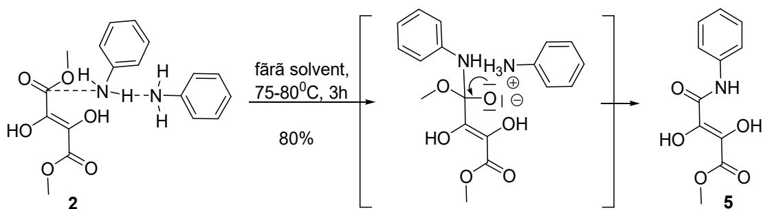
Fig. 3.3. Schema de sinteză a ( E )-metil 2,3-dihidroxi-4-oxo-4-(fenilamino)but-2-enoatului 5
