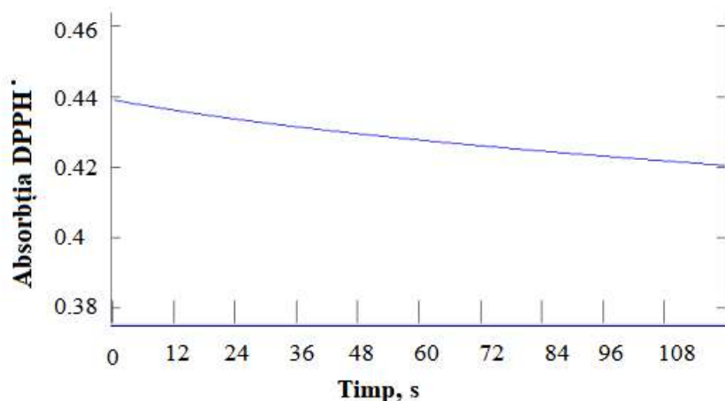
Fig. 3.27. Scăderea absorbției radicalului DPPH • în timp, la interacțiunea cu anilida 5 , în primele 120 secunde de reacție, pentru condiția [anilida]_0 = [DPPH^{\bullet}]_0/\sigma
