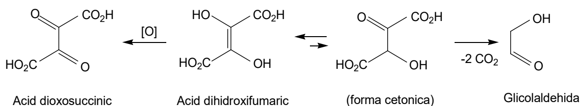
Fig. 1.2. Prezentarea schematică a principalelor căi de degradare a DFH 4 în soluție
