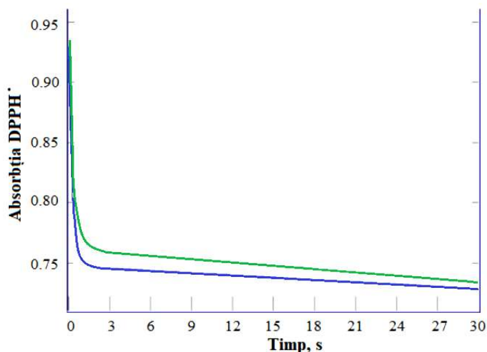
Fig. 3.11. Curbele cinetice de consum a DPPH • la interacțiunea cu DFH 4 1 (albastru) și acidul MBD 12 (verde) în condițiile: [DFH 4 ] 0 = [MBD] 0 = 2·10 -5 M; [DPPH • ] 0 = 1·10 -4 M, t = 30 s
