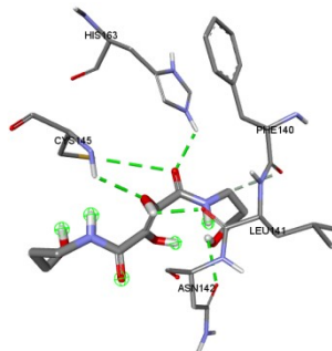
Fig. 4.21. Reprezentarea interacțiunii cu cel mai mare scor de andocare între compusul cercetat și proteaza principală a virusului SARS-COV-2 (imagine 3D - pe stânga și 2D - pe dreapta), pentru substanțele cercetate: (a) anilida 5, (b) fumaramida 6, (c) MEAD 7, (d) MPAD 8
