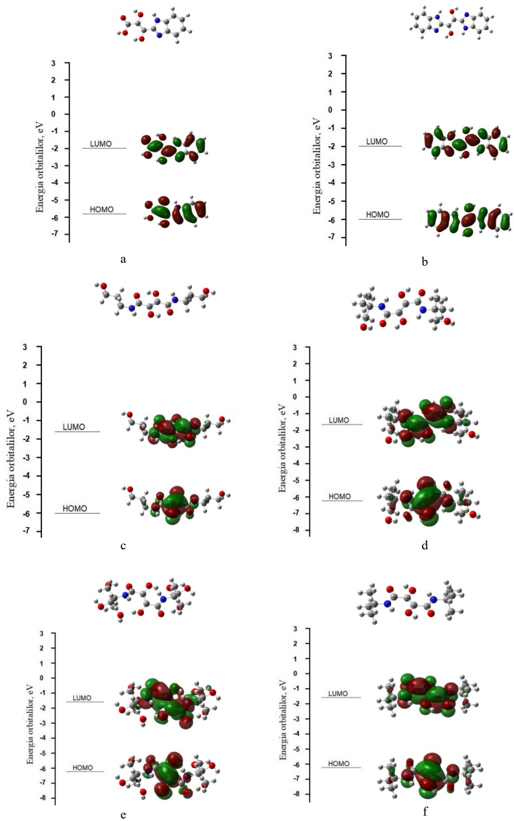
Fig. 4.15. Energia orbitalilor și unii orbitali moleculari de frontieră pentru (a) MBD 12, (b) BBD 13, (c) MPAD 8, (d) fumaramida 9, (e) fumaramida 10, (f) fumaramida 11
