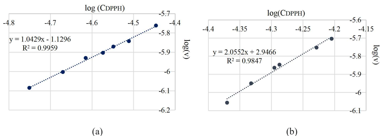
Fig. 3.26. Determinarea ordinului de reacție x față de DPPH • (a), și a ordinului total de reacție x+y (b) în reacția radicalului DPPH • cu esterul EMD 2 , unde [EMD]_0 = 2 \cdot 10^{-5} \text{ M} (a) și [EMD]_0 = [DPPH^{\bullet}]_0 (b), timpul de reacție t = 1 \text{ s}
