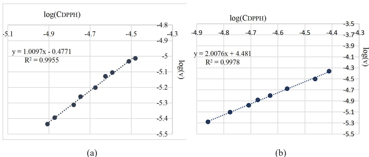
Fig. 3.24. Determinarea ordinului de reacție x față de DPPH' (a), și a ordinului total de reacție x+y (b) în reacția radicalului DPPH' cu BBD 13, unde [BBD]_0 = 2 \cdot 10^{-5} \text{ M} (a) și [BBD]_0 = [DPPH']_0/\sigma , unde \sigma = 1 (b), la timpul de reacție t = 0.2 \text{ s}
