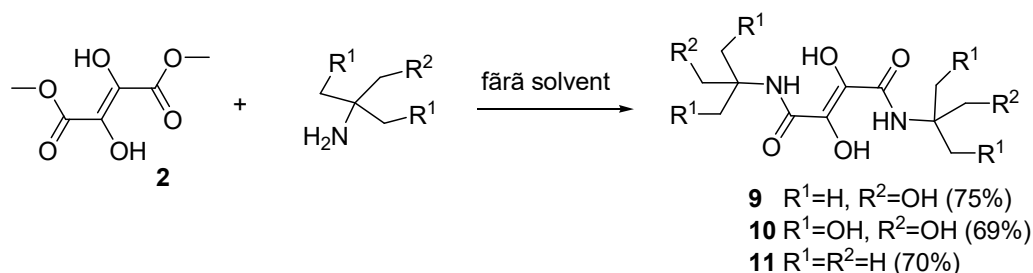
Fig. 3.7. Schema de sinteză a 2,3-dihidroxi-N1,N4-bis(1-hidroxi-2-metilpropan-2-il)fumaramidei 9 , N1,N4-bis(1,3-dihidroxi-2-(hidroximetil)propan-2-il)-2,3-dihidroxifumaramidei 10 și N1,N4-di-tert-butil-2,3-dihidroxifumaramidei 11
