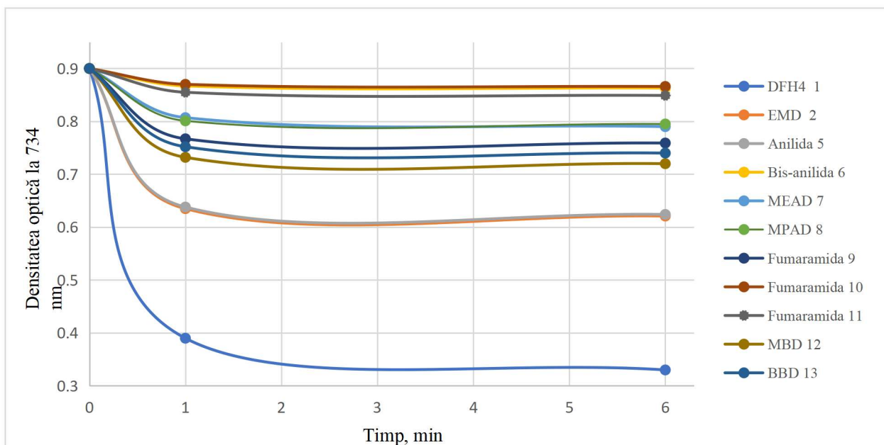
Fig. 3.30. Descreșterea absorbției soluțiilor de ABTS ++ în funcție de natura reducătorilor, pentru [Red] 0 = 25 μM
