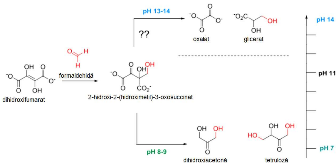
Fig. 1.16. Reprezentarea schematică a divergenței datorate pH-ului pentru reacția dintre dihidroxifumarat și formaldehidă [60]
