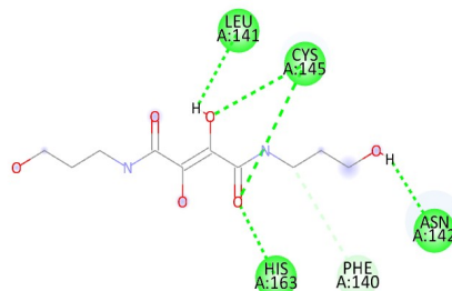
Fig. 4.21. Reprezentarea interacțiunii cu cel mai mare scor de andocare între compusul cercetat și proteaza principală a virusului SARS-COV-2 (imagine 3D - pe stânga și 2D - pe dreapta), pentru substanțele cercetate: (a) anilida 5, (b) fumaramida 6, (c) MEAD 7, (d) MPAD 8
