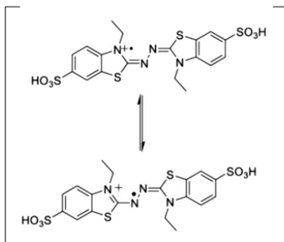
Fig. 2.3. Structura moleculară a radicalului ABTS •+
