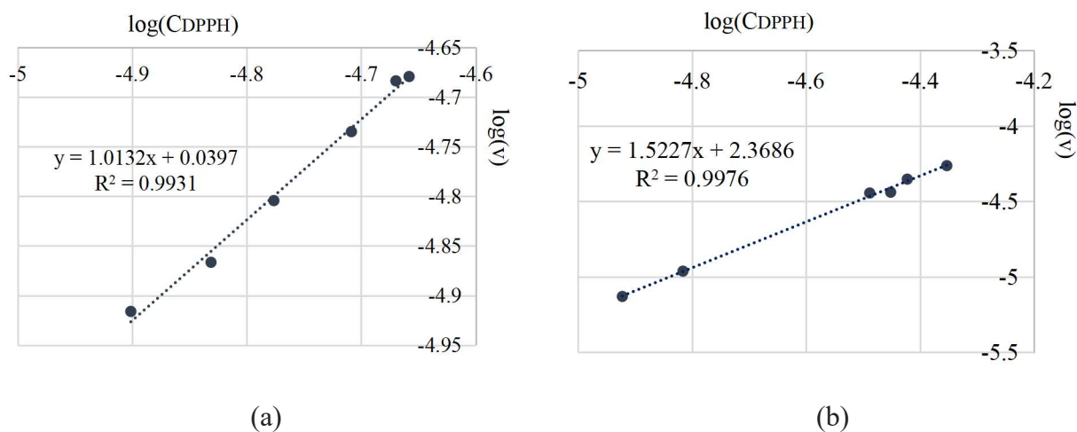
Fig. 3.18. Determinarea ordinului de reacție x față de DPPH^* (a), și a ordinului total de reacție x+y (b) în reacția radicalului DPPH^* cu AAs, unde [AAs]_0 = 2 \cdot 10^{-5} M (a) și [AAs]_0 = [DPPH^*]_0/\sigma (b), la timpul de reacție t = 0.2 s
