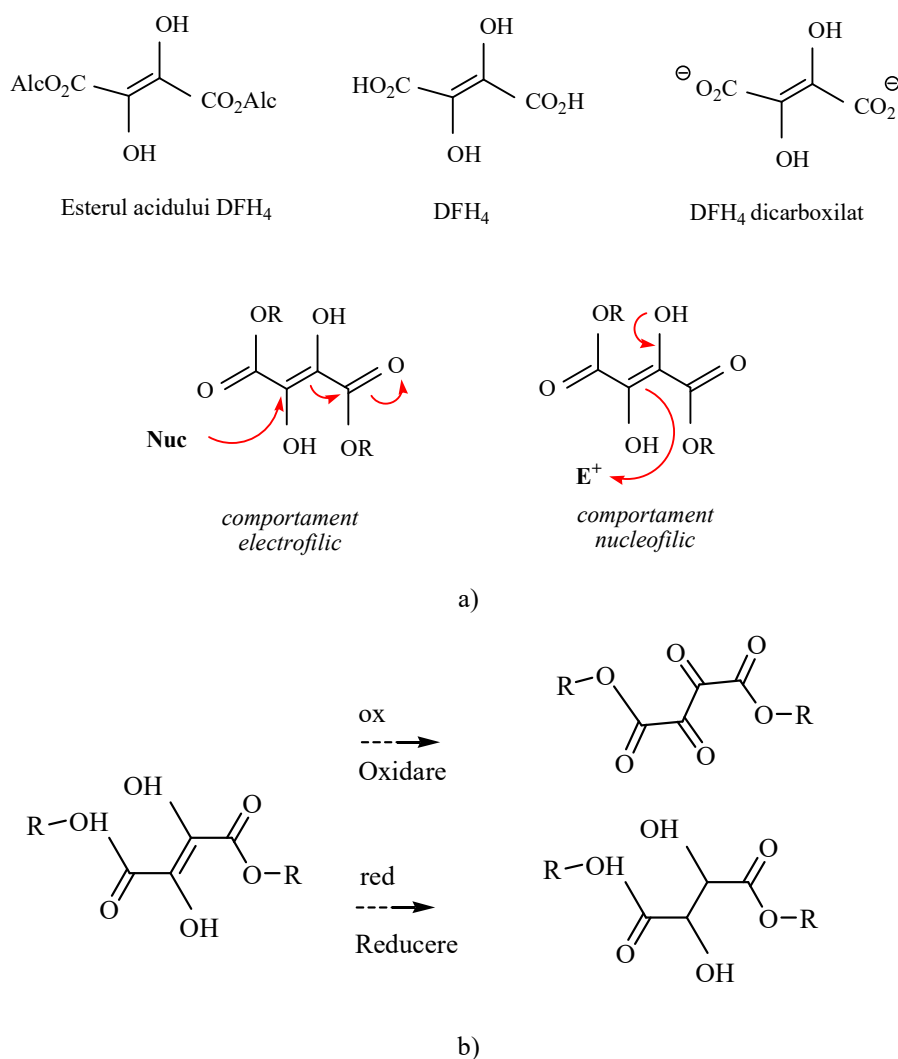
Fig. 1.3. Reprezentarea schematică a electrofilicității și nucleofilicității DFH 4 (a) și a caracterului oxidant/reducător (b) [38]
