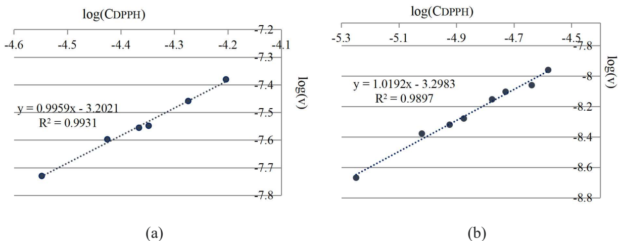
Fig. 3.28. Determinarea ordinului de reacție x față de DPPH • (a), și a ordinului de reacție y (b) față de anilida 5 , unde [anilida]_0 = 2,26 \cdot 10^{-5} \text{ M} (a) și [DPPH^{\bullet}]_0 = 2 \cdot 10^{-5} \text{ M} (b), timpul de reacție t = 10 \text{ min}
