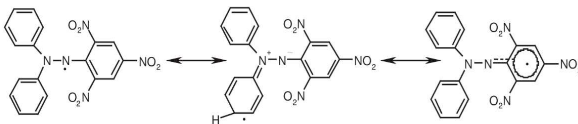
Fig. 2.1. Structura moleculară a radicalului stabil de DPPH*
