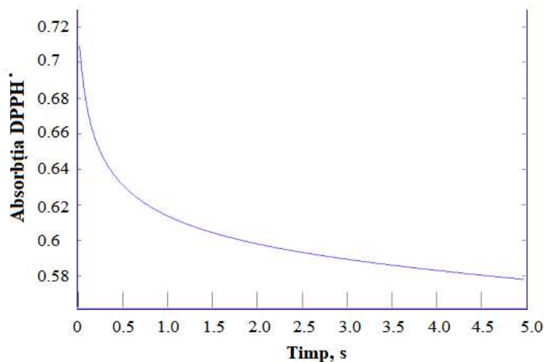
Fig. 3.23. Scăderea absorbției radicalului DPPH' în timp, la interacțiunea cu BBD 13, în primele 5 secunde de reacție, pentru condiția [BBD]_0 = [DPPH']_0/\sigma , unde \sigma = 1
