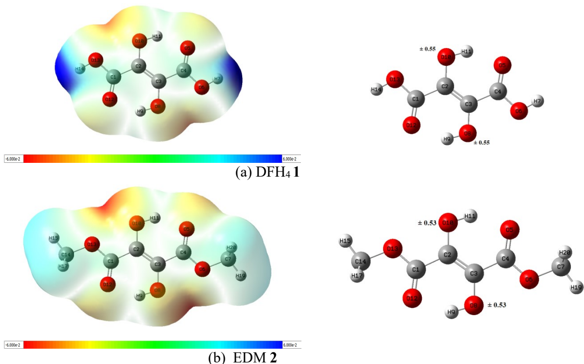
Fig. 4.7. Hărțile MEP (pe stânga) și indicele ambifilic R_k (pe dreapta) ale DFH4 1 și EDM 2, în metanol
