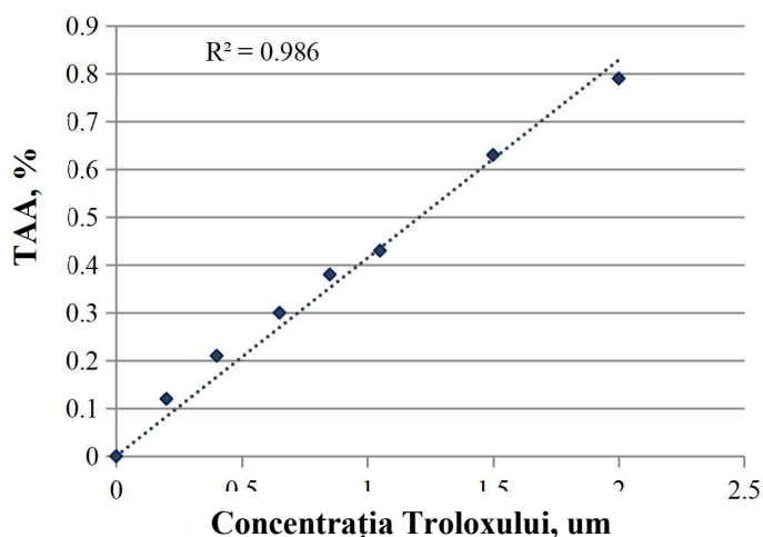
Fig. 3.29. Activitatea antioxidantă totală a soluției de Trolox, în funcție de [Trolox] 0 , determinată prin metoda ABTS •+
