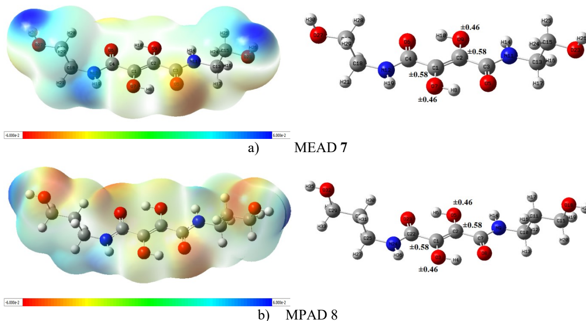
Fig. 4.10. Hărțile MEP (pe stânga) și indicele ambifilic R_k (pe dreapta) ale MEAD 7 (a) și MPAD 8 (b), în metanol
