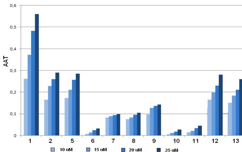
Fig. 3.31. Dependența AAT de natura și concentrația reducătorilor
