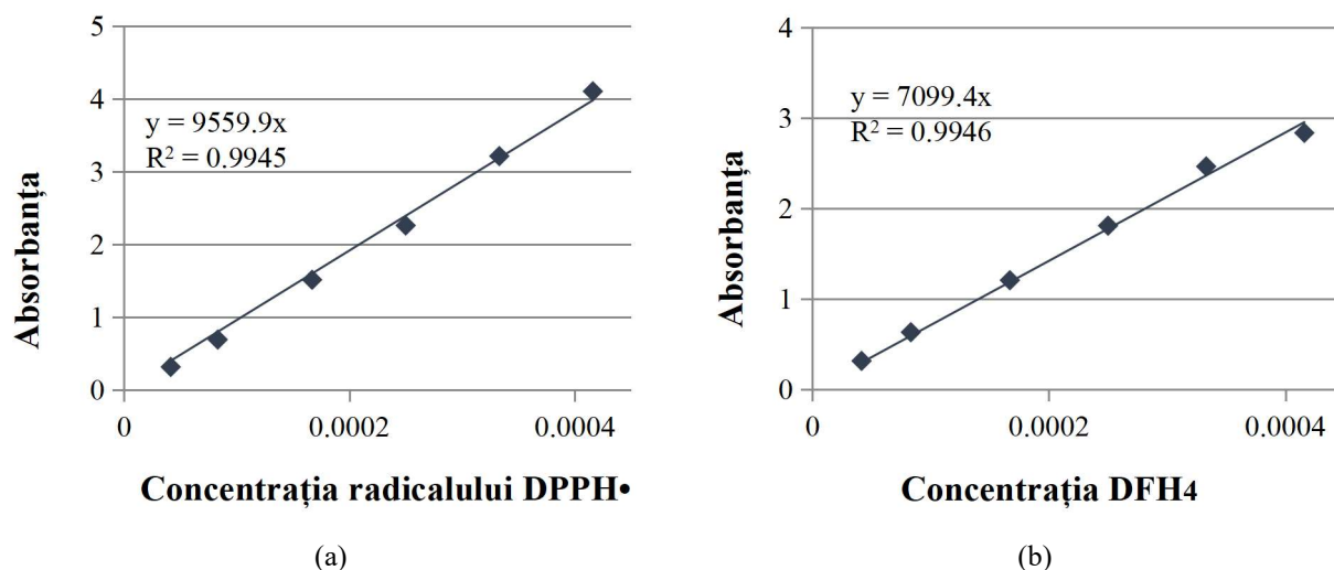
Fig. 3.9. Curbele de calibrare pentru DPPH• (a) și DFH4 (b) în soluție metanolică (70%)
