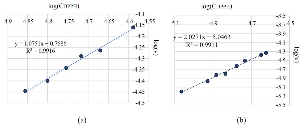
Fig. 3.22. Determinarea ordinului de reacție x față de DPPH• (a), și a ordinului total de reacție x+y (b) în reacția radicalului DPPH• cu MBD 12, unde [MBD]_0 = 2 \cdot 10^{-5} \text{ M} (a) și [MBD]_0 = [DPPH•]_0/\sigma , unde \sigma = 2 (b), la timpul de reacție t = 0.2 \text{ s}
