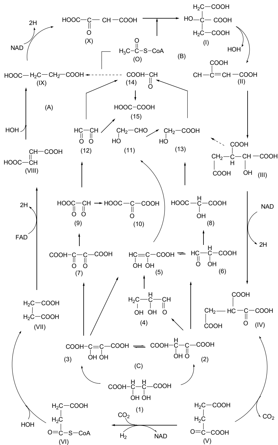
Fig. 1.11. Interrelația ciclurilor metabolice [50]
