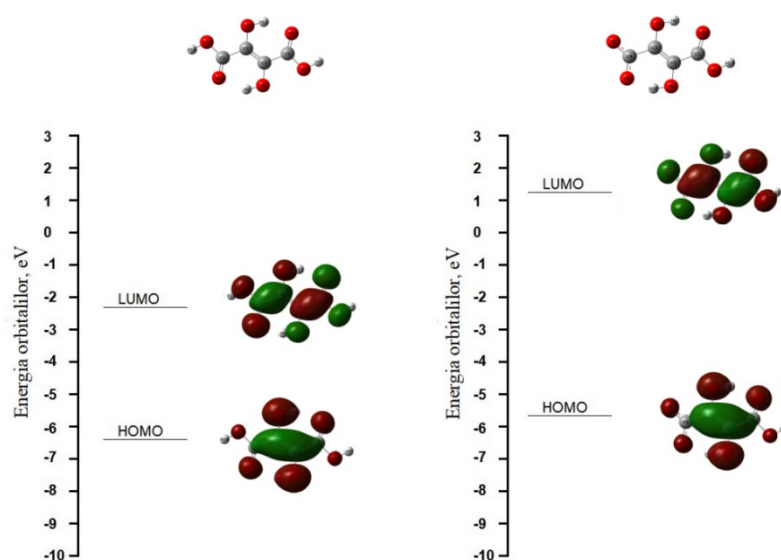
Fig. 4.13. Energia orbitalilor și unii orbitali moleculari de frontieră ai izomerului E3 (stânga) al acidului DFH 4 și anionul respectiv
