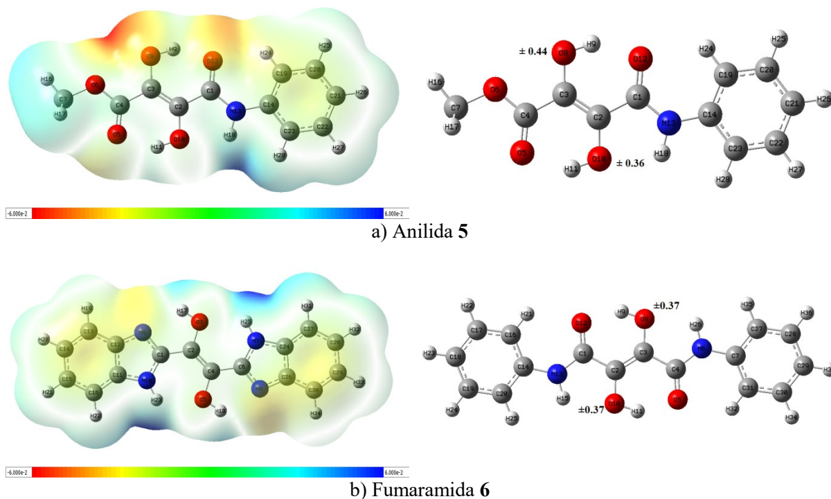
Fig. 4.8. Hărțile MEP (pe stânga) și indicele ambifilic R_k (pe dreapta) ale anilidei 5 și fumaramidei 6, în metanol
