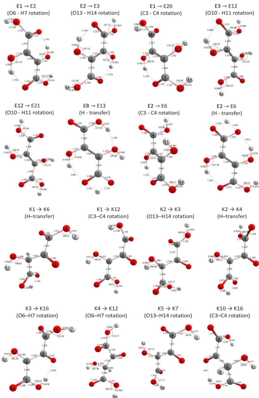
Fig. 4.4. Structurile geometrice optimizate ale unor ST caracteristice pentru interconversiile enediol-enediol și cetonă-cetonă, în apă
