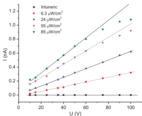
Fig.3. Dependenta I-U la iluminări din intervalul densităților de flux 6-85 \mu\text{W}/\text{cm}^2
