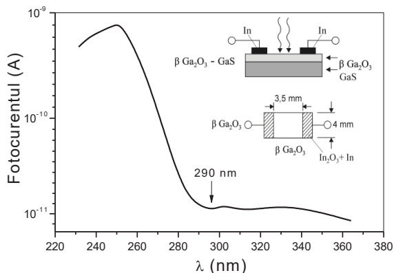
Fig.4. Dependenta spectrală a curentului în fotorezistorul pe baza stratului subțire de \beta\text{-Ga}_2\text{O}_3
