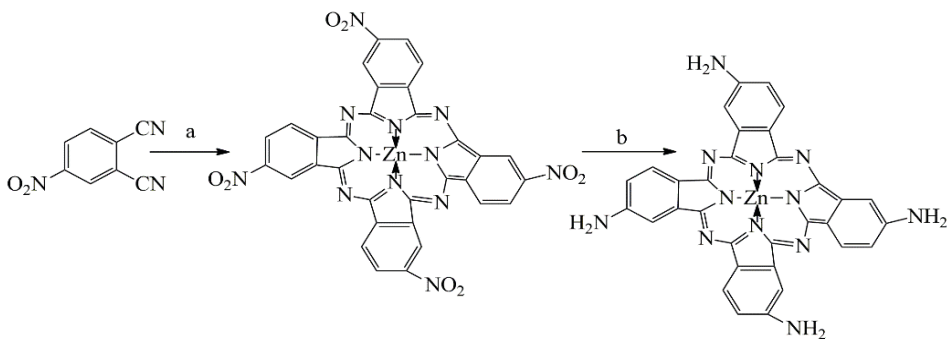
Fig. 1. Sinteza ftalocianinelor de Zn substituite cu grupe -\text{NO}_2 și -\text{NH}_2 .
