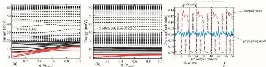
Рис. 1. Фононные спектры в кремниевых нанонитях и среднеквадратические смещения атомов [8]. (а) поперечное сечение нити 14 монослоев (МС) x 14 монослоев; (б) поперечное сечение узких сегментов нити 14 МС x 14 МС, широких - 22 МС x 22 МС, длина сегментов N_z = 6МС ; (в) красная линия – захваченная мода, синяя линия – общая мода
