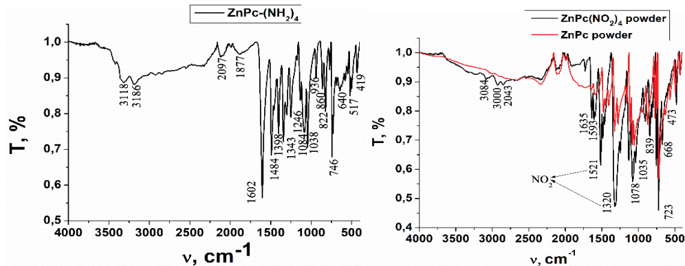
Fig. 2. Spectrele FTIR ale ftalocianinei de Zn substituite cu grupe -\text{NH}_2 ( \text{ZnPc}(\text{NH}_2)_4 stânga) și grupe -\text{NO}_2 ( \text{ZnPc}(\text{NO}_2)_4 dreapta).
