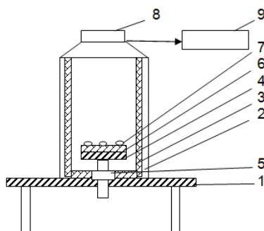
Fig. 3. Instalația pentru tratarea semințelor cu frecvențe acustice [15, p. 34]: 1 – suport fix; 2 – cilindru; 3 – strat absorbant; 4 – suport mobil; 5 – șurub; 6 – suport; 7 – semințe supuse tratamentului; 8 – difuzor; 9 – generator de sunete.
