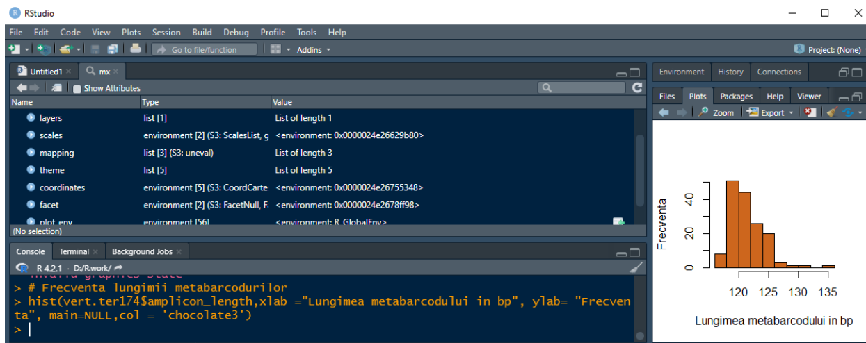
Fig. 2.6. Utilizarea RStudio pentru reprezentarea grafică a frecvenței lungimii metabarcodurilor [167]
