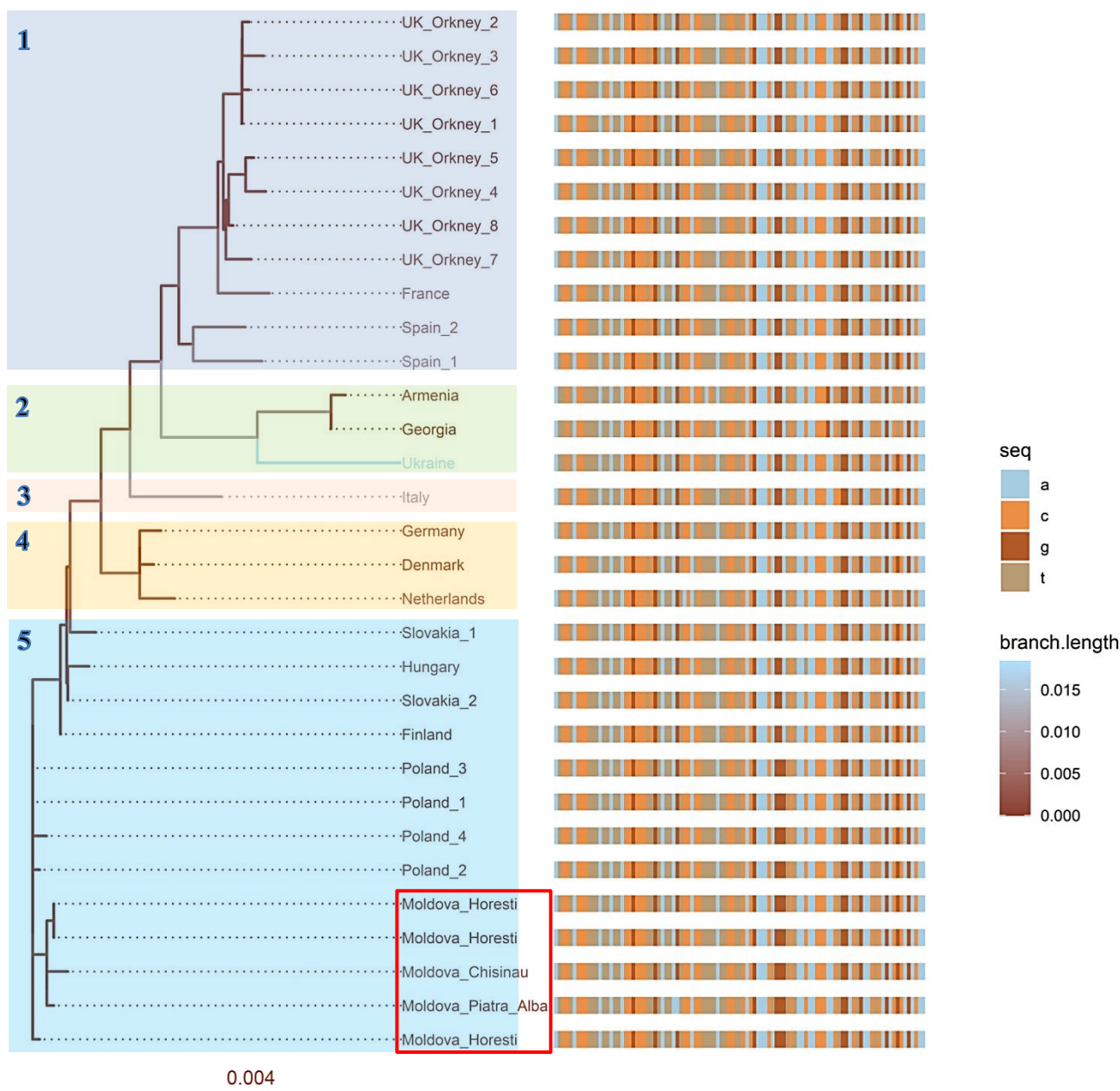
Fig. 4.3. Arborele filogenetic obținut din secvențe ale genei CYTB la specia M. arvalis
