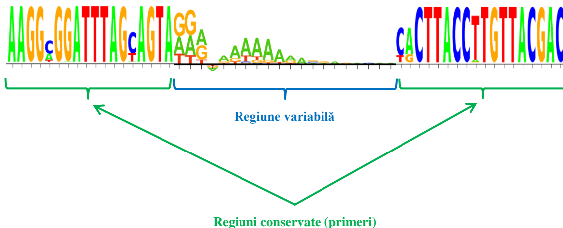
Fig. 1.2. Structura unui metabarcod [159]
