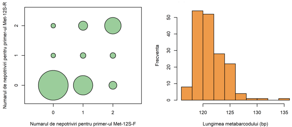
Fig. 3.7. Numărul de nepotriviri (stânga) și lungimea metabarcodurilor (dreapta) pentru perechea de primeri Met-12S
