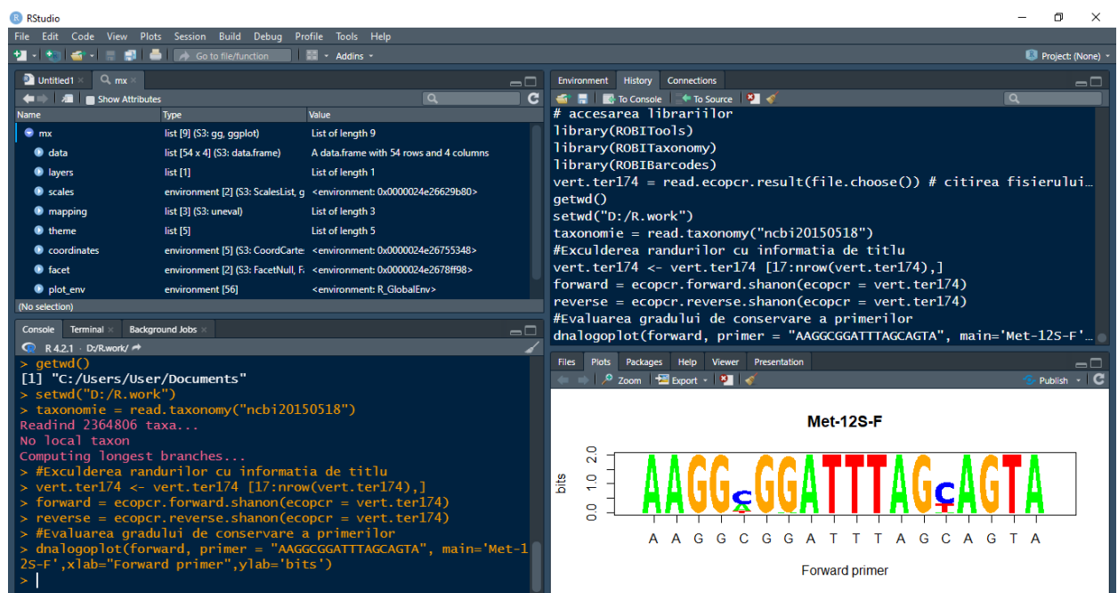
Fig. 2.4. Evaluarea gradului de conservare a primerilor (mediul Rstudio)
