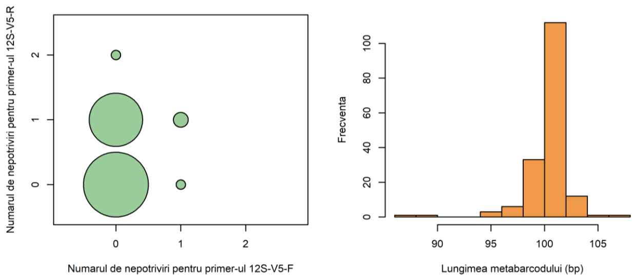
Fig. 3.8. Numărul de nepotriviri (stânga) și lungimea metabarcodurilor (dreapta) pentru perechea de primeri 12S-V5
