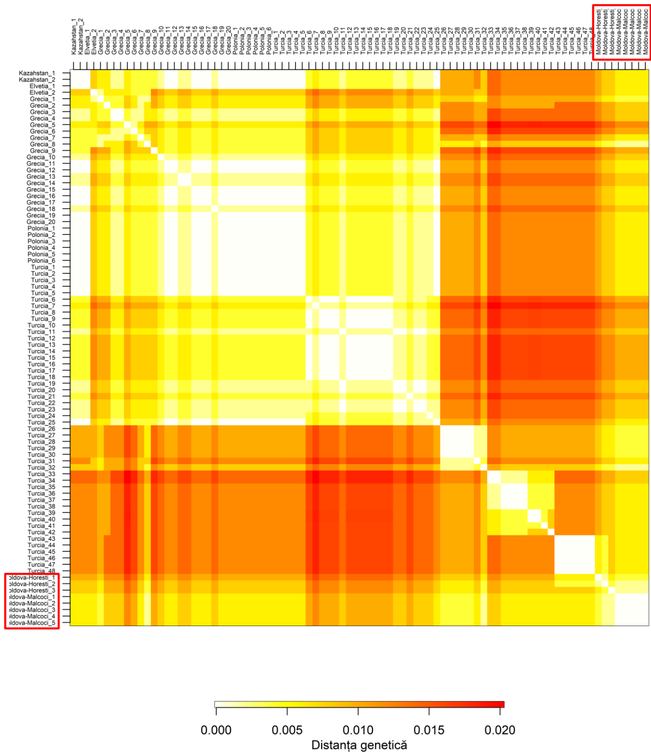
Fig. 4.5. Distanța genetică între 86 secvențe ale geni CYTB la specia M. levis
