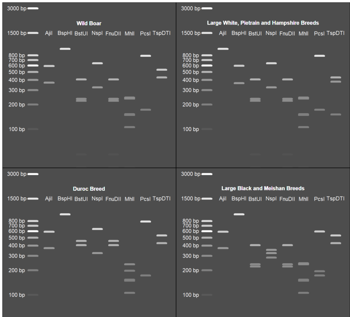
Fig. 3.9. Electroforegrama obținută în urma simulării digestiei secvențelor alelice MC1R Enzime de restricție utilizate – AjiI , BspHI , BstUI , NspI , FnuDII , MhII , PcsI , TspDTI
