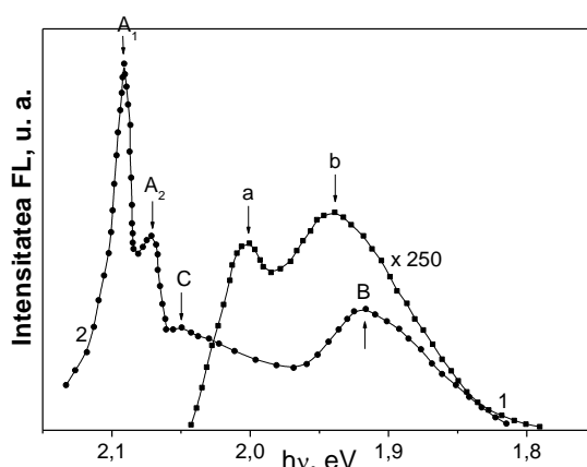
Fig. 2. Spectrele de fotoluminescență ale cristalelor \epsilon\text{-GaSe} la temperatura 300 K (curba 1) și la temperatura 78 K (curba 2). Excitare cu \lambda = 337,4 \text{ nm} , densitatea energetică \sim 100 \text{ mW/cm}^2
