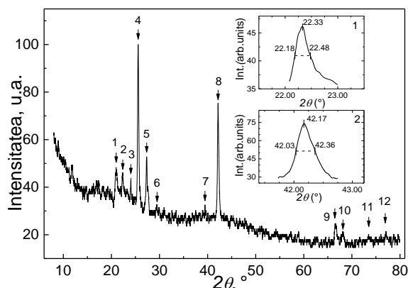
Fig. 1. Difractograma XRD a compusului GaSe intercalat cu Cd la temperatura 753 K.
