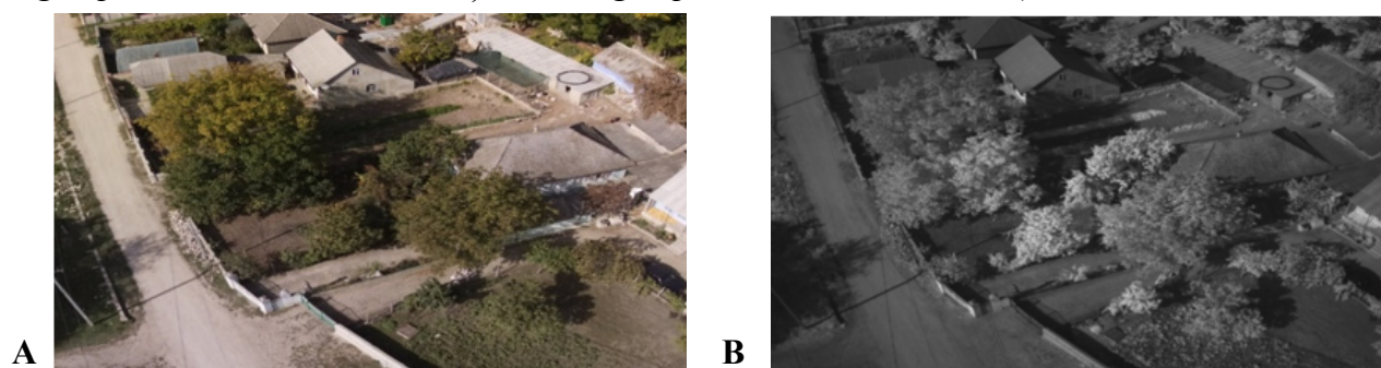
Figura 1. Determinarea stării de sănătate a plantelor cu ajutorul aparatului multispectral (A – imagini prelevate cu camera RGB și B – imagini prelevate cu camera NIR).
